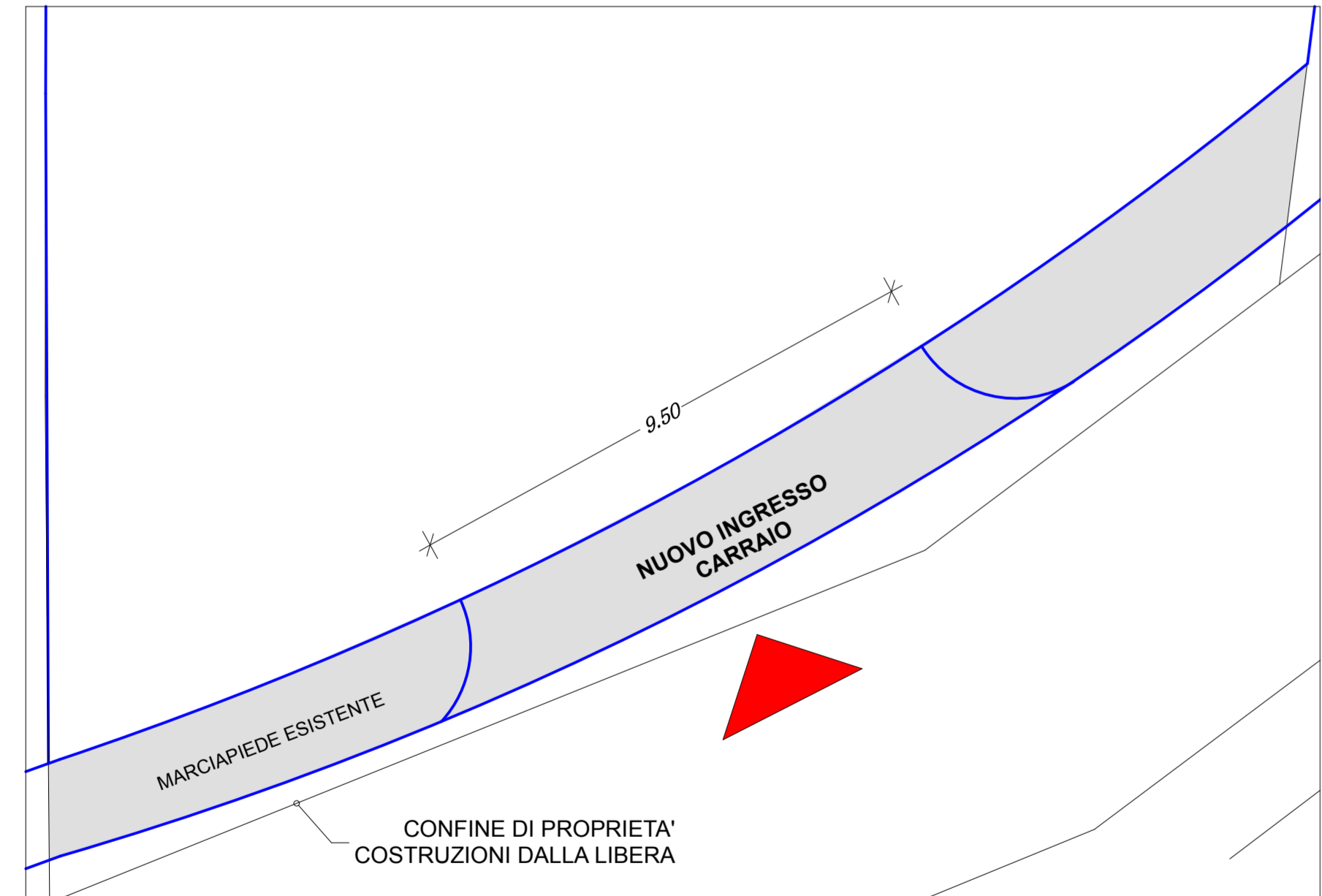
PARTICOLARE NUOVO INGRESSO CARRAIO 1:100
